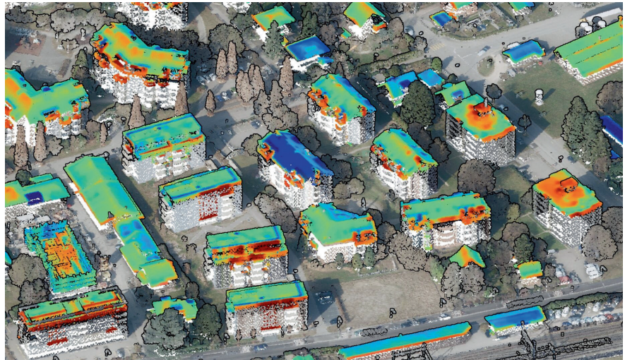
Bild 1 Hochaufgelöste Thermalaufnahme der Dächer zeigen die Wärmeabstrahlung von blau (kälter) bis rot (wärmer) auf dem Hintergrund eines 3D-Oberflächenmodells (aus Lidar-Daten) eingefärbt mit Information aus RGB-Luftbildern.
